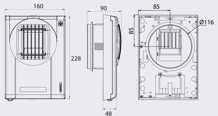
Méretetek (mm)
